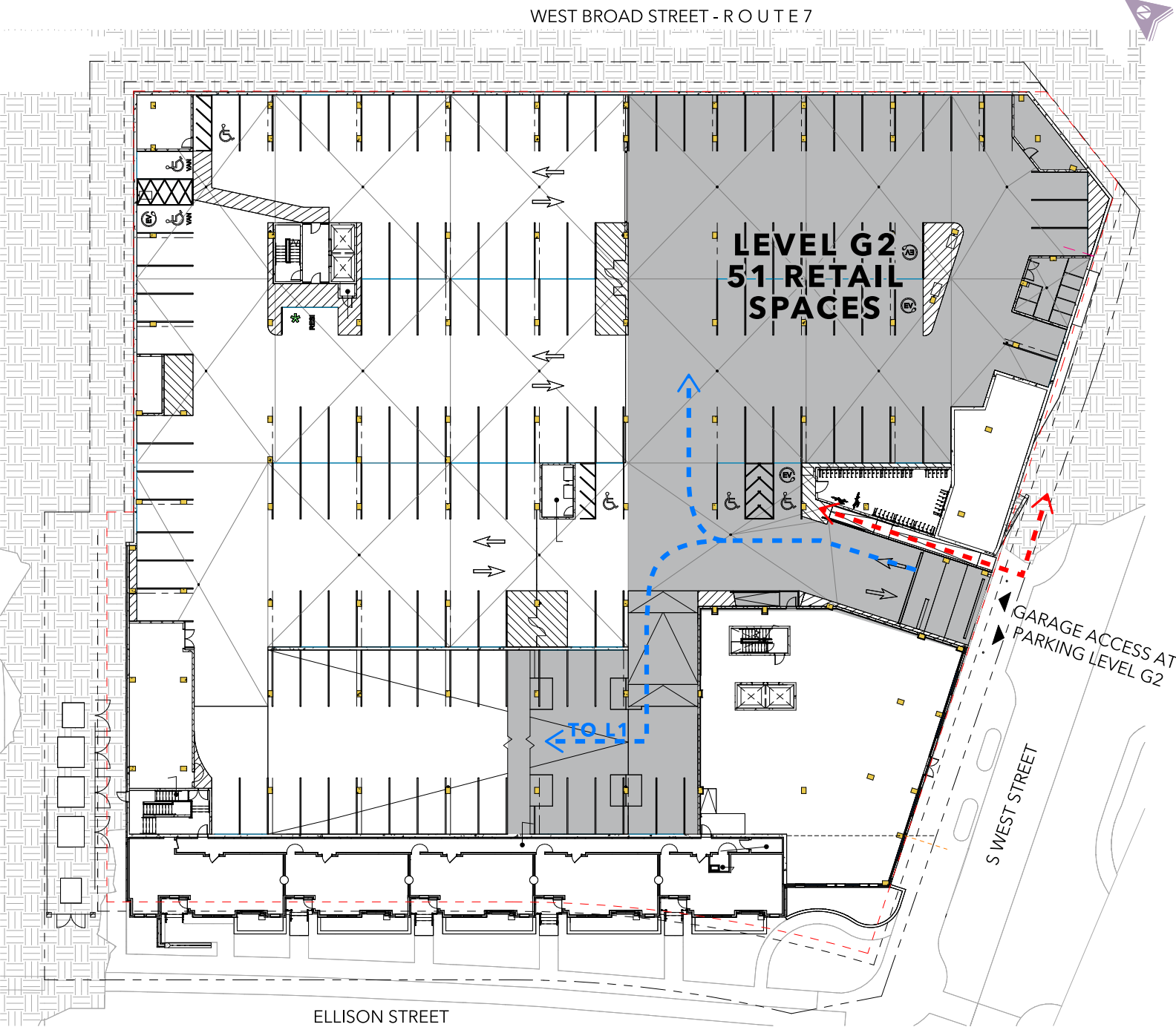
LEVEL G2
